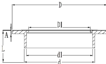
管固定座 Beam Fittings 單位：mm
